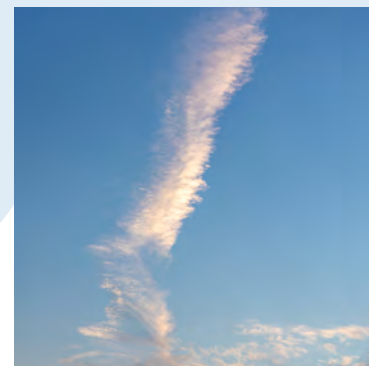
Cirrus fibratus
