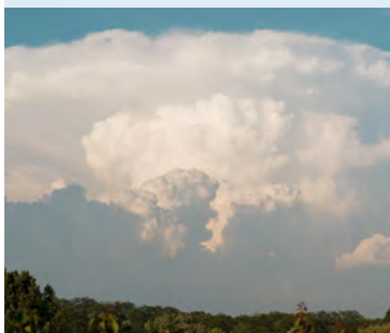
Cumulus congestus
