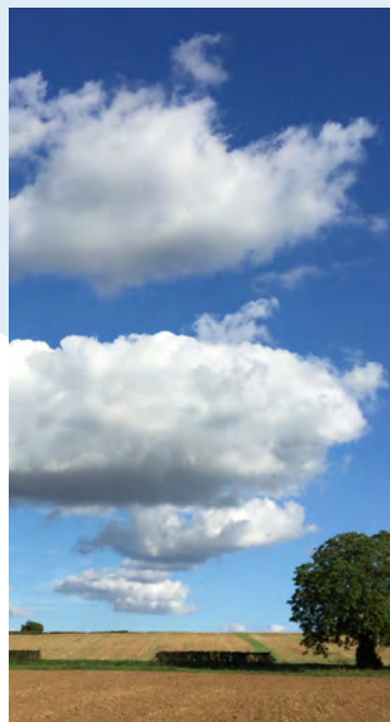
Cumulus humilis
