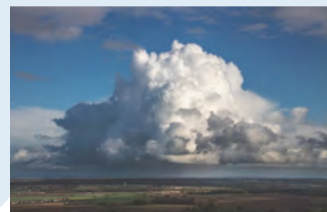
Cumulus mediocris
